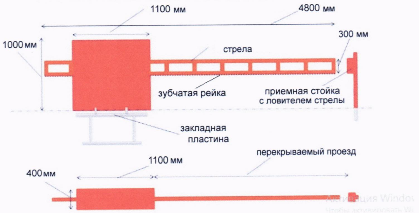
Рис. 1. Размеры шлагбаума
